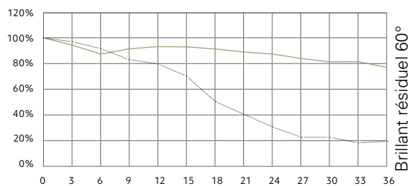
Durée d'exposition (mois) — RAL 5010 .....Standard
